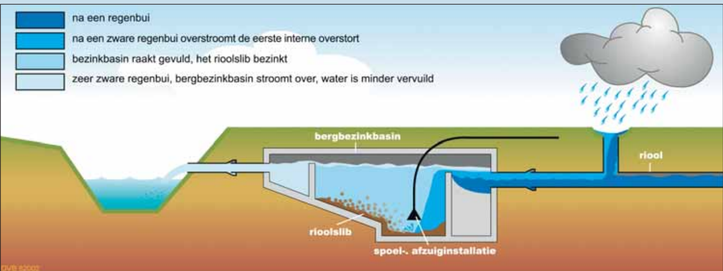
Riooloverstort met bergbezinkbassin
