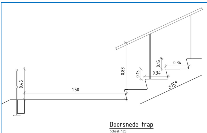
Trap in talud met visplateau
